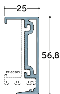
TV 80402 6,5m 845 gr/m Interlock Profile 25mm
