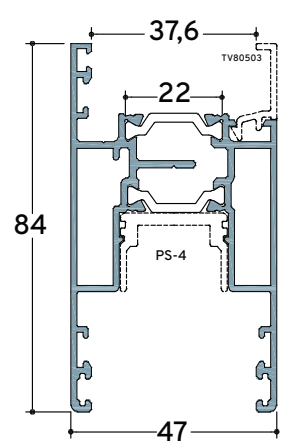
TV 80402 6,5m 845 gr/m Interlock Profile 25mm
